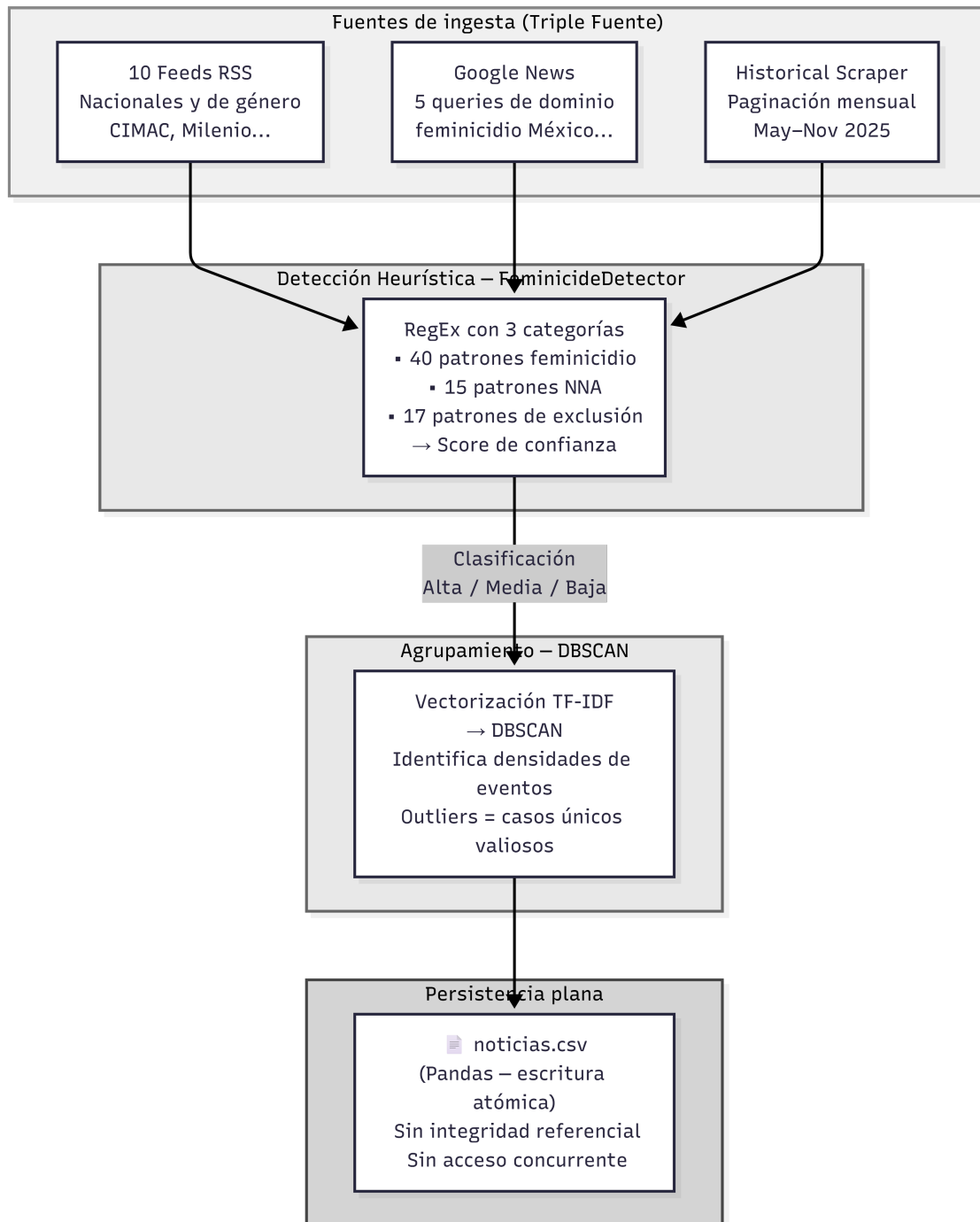
Figura 6.1: Diagrama de flujo del prototipo 2.
