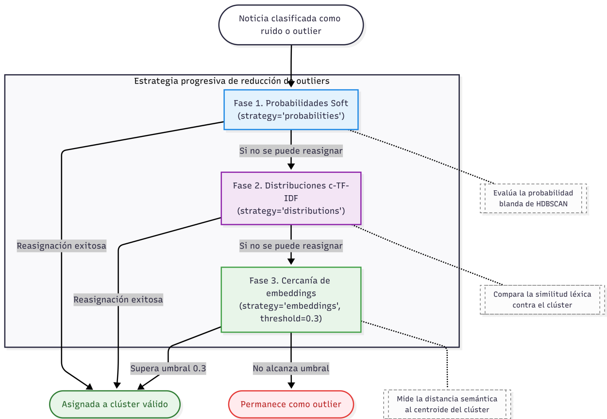
Figura 3.3: Reducción de outliers en BERTopic
