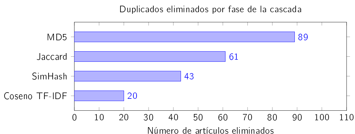
Figura 8.1: Distribución de duplicados eliminados por fase de la cascada de deduplicación.
