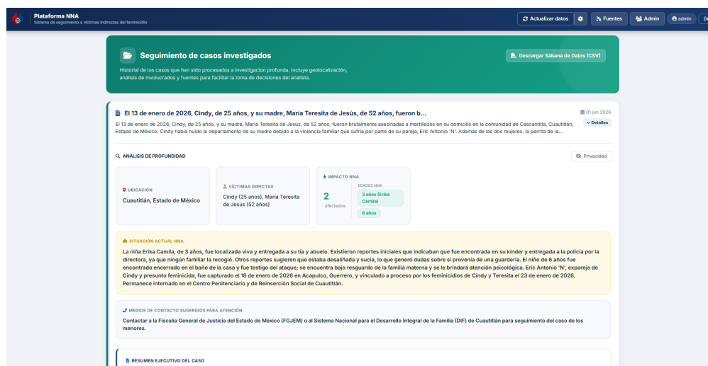
Figura 5.4: IU-04 Pantalla de Seguimiento de Casos Activos.
