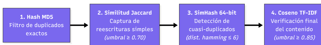
Figura 7.3: Flujo de deduplicación en cascada.
