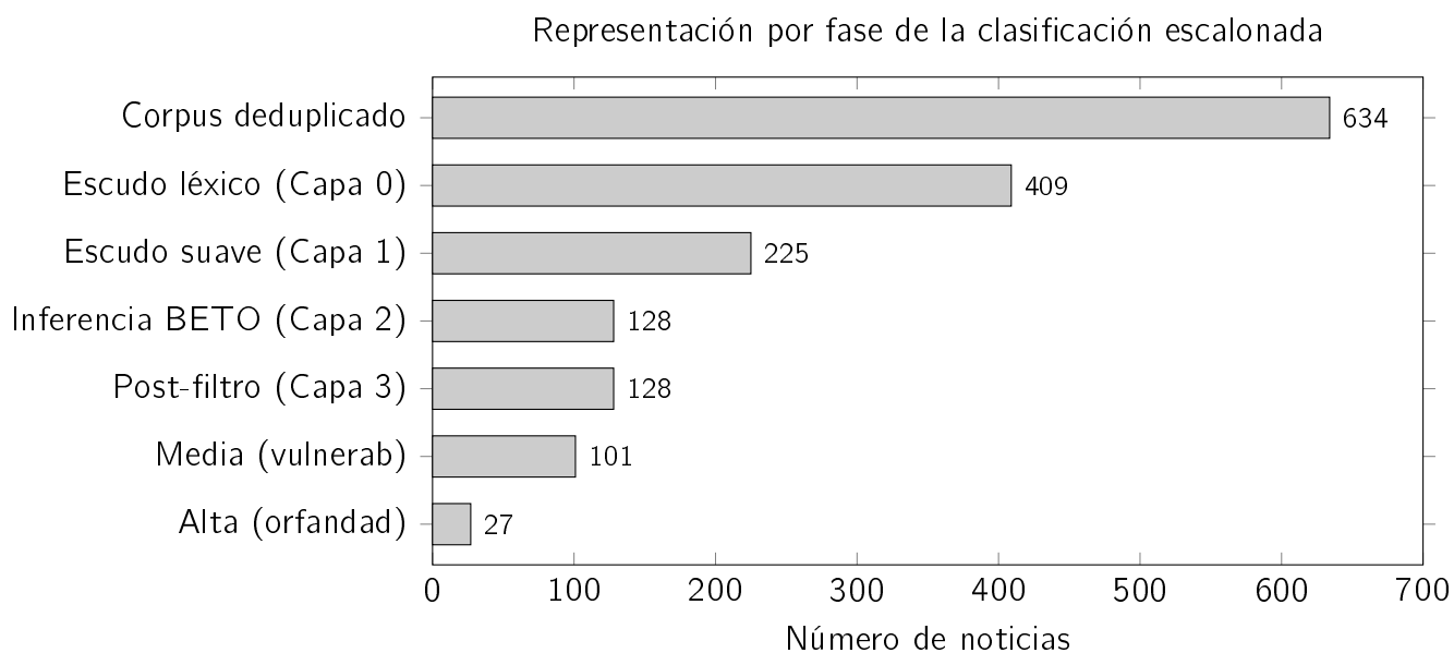
Figura 8.2: Reducción del corpus desde 634 noticias únicas hasta 27 casos de alta relevancia.
