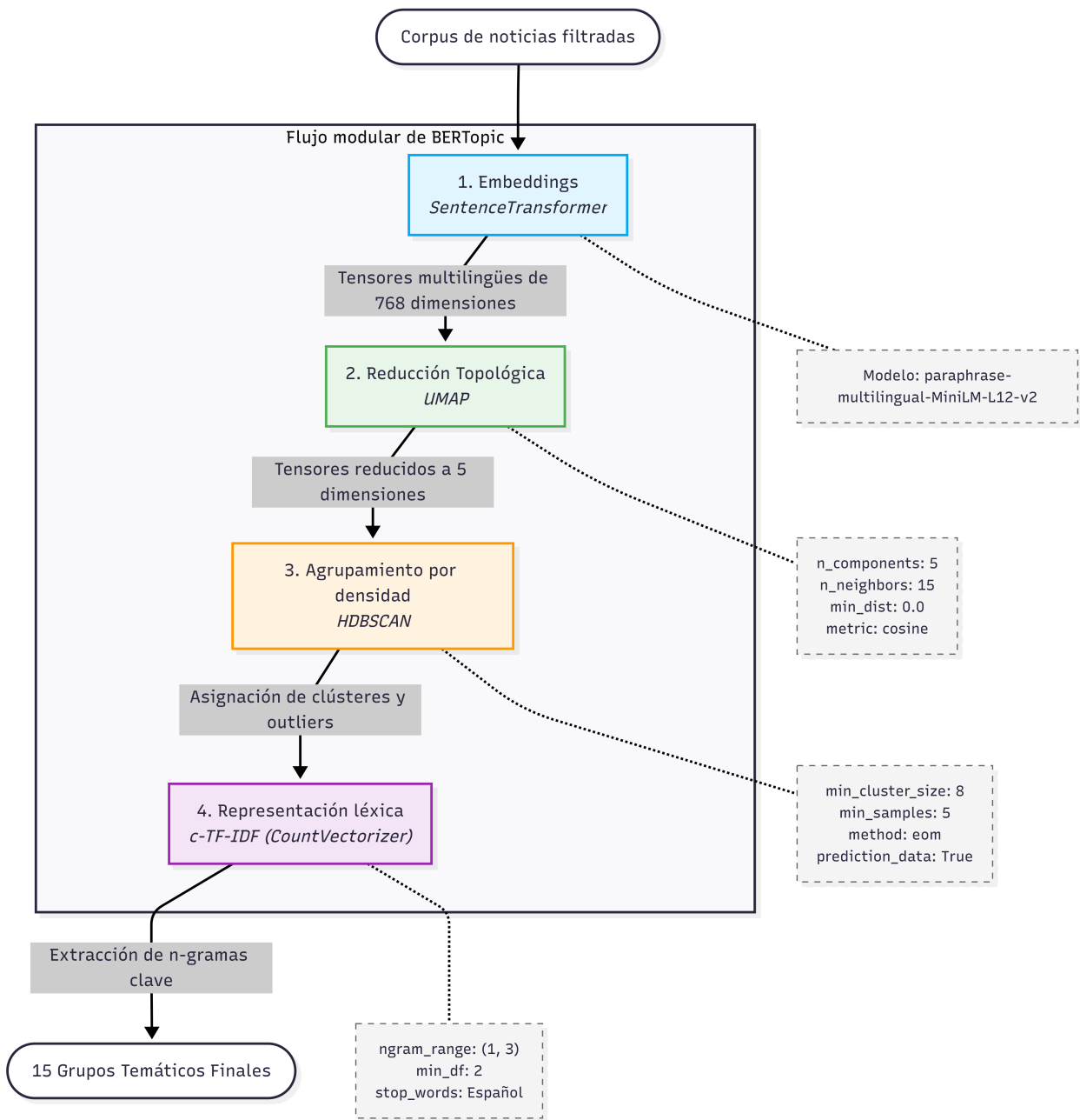
Figura 3.2: Arquitectura modular de BERTopic y su parametrización en TT II
