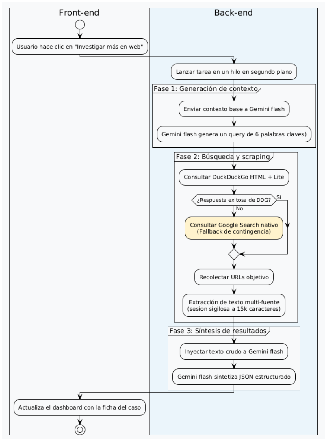
Figura 7.4: Flujo de investigación profunda.
