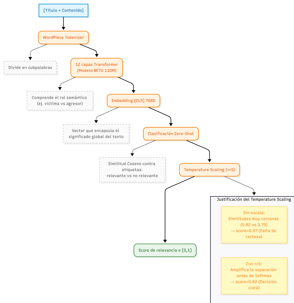
Figura 7.2: Arquitectura del motor BETO y clasificación Zero-Shot con Temperature Scaling .
