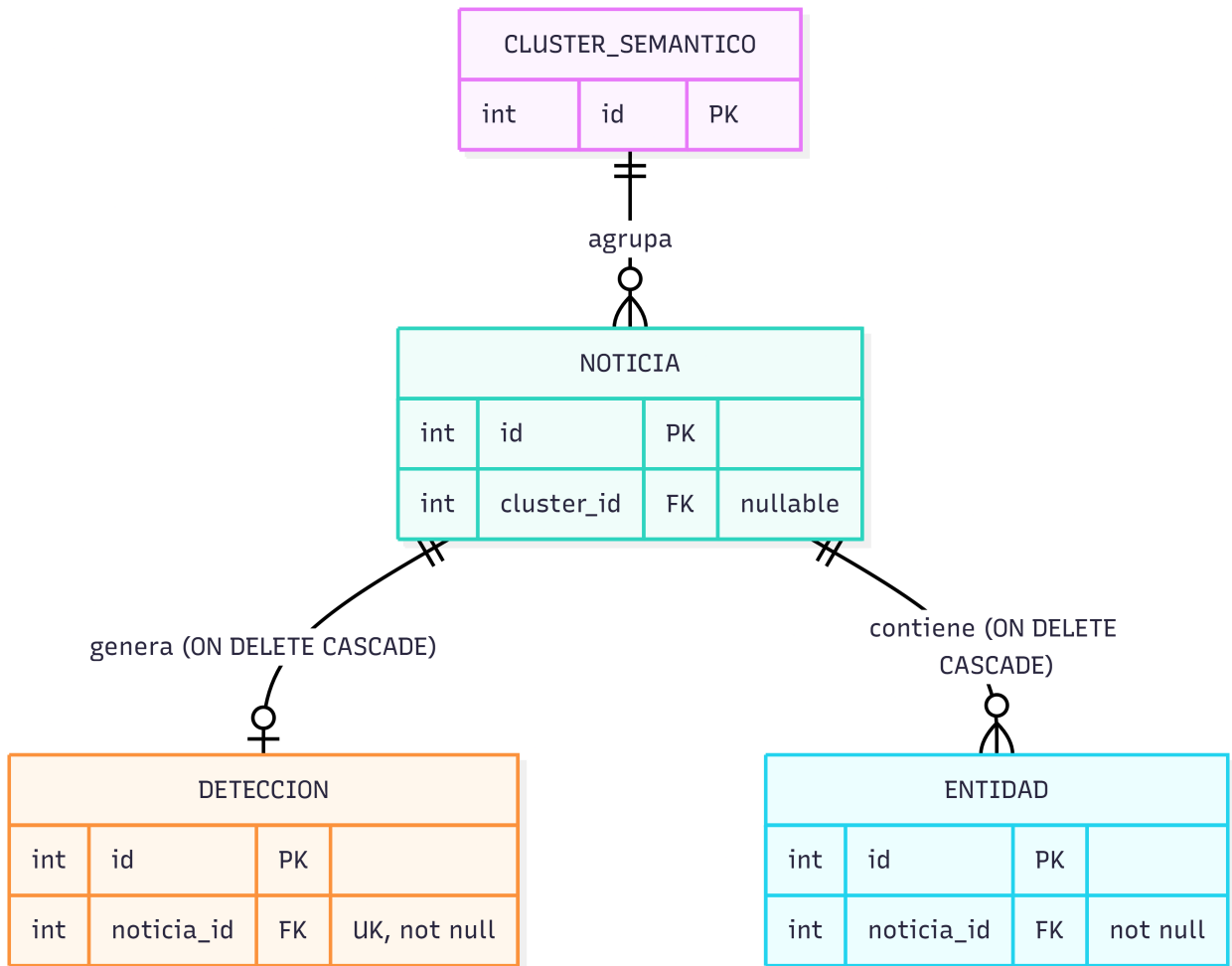
Figura 3.1: Esquema relacional
