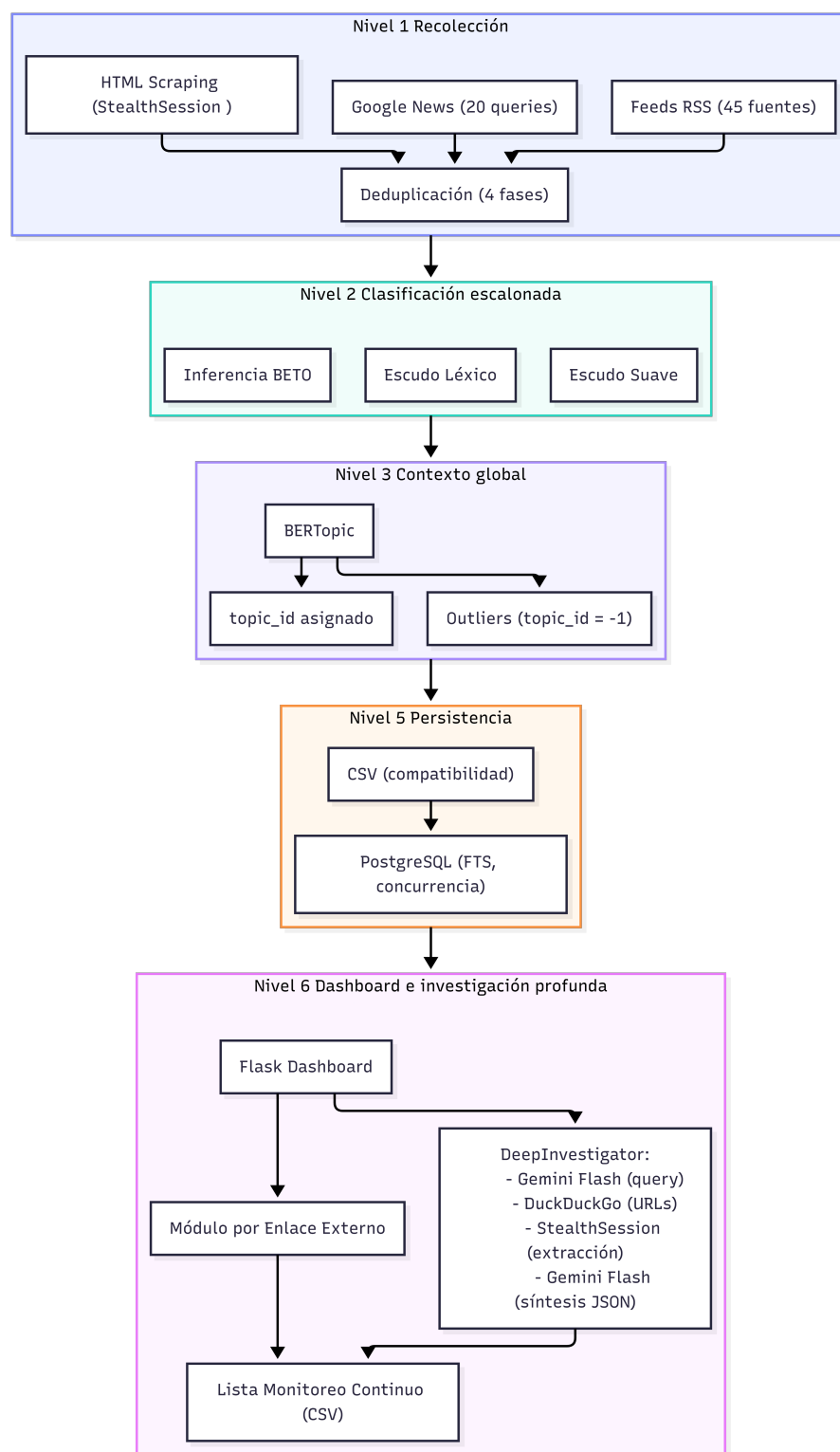
Figura 7.5: Arquitectura del Sistema de Clasificación Escalonada.
