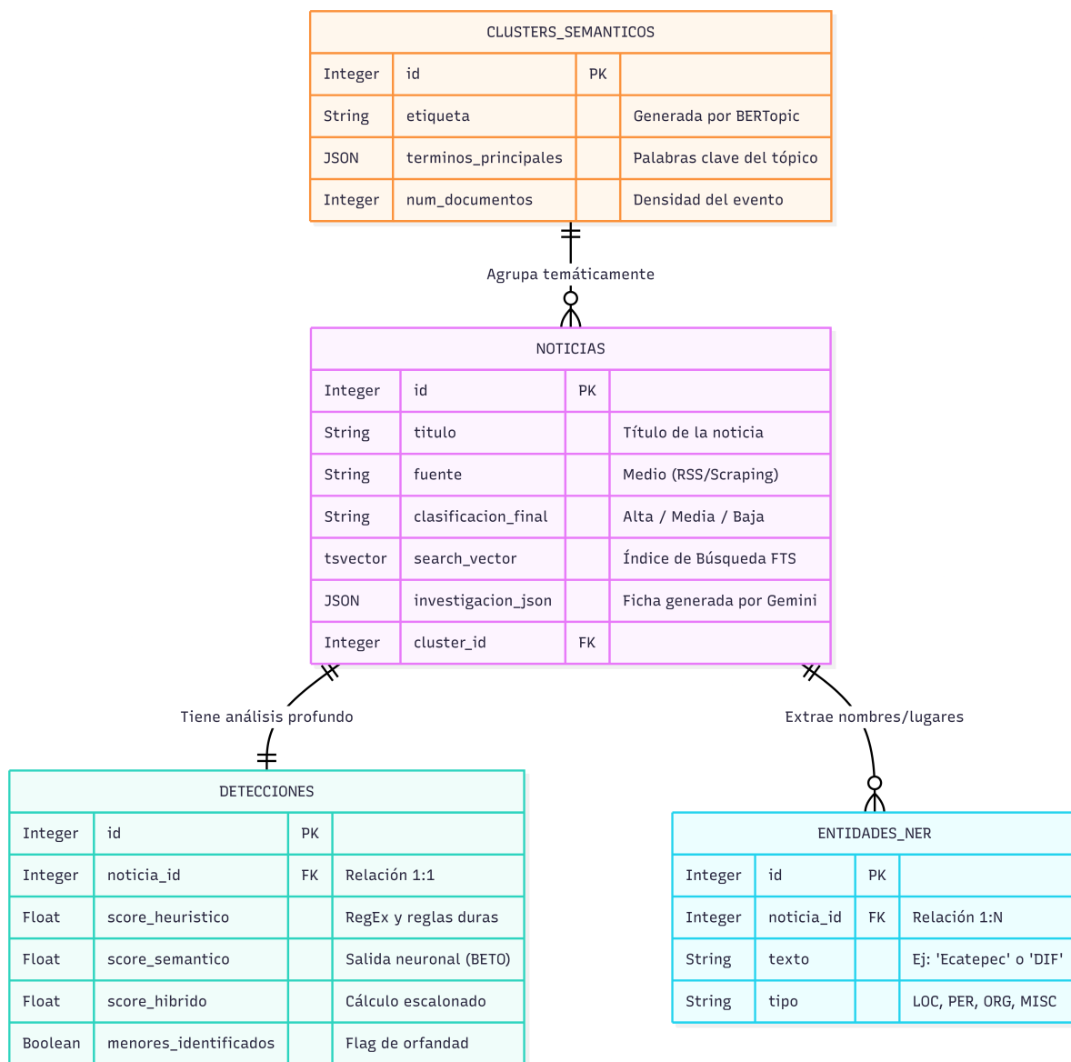
Figura 7.1: Modelo entidad-relación de la base de datos en PostgreSQL.
