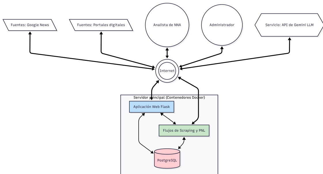
Figura 4.2: Arquitectura del sistema.
